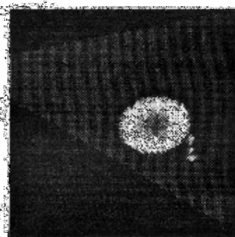
(f) Otsu 法 (13.4)
